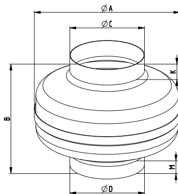
Рисунок 1. Габаритные и присоединительные размеры
