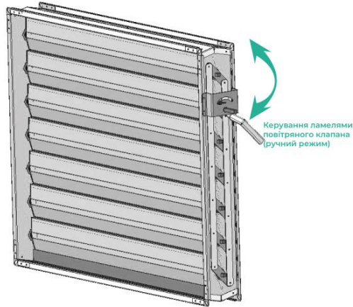
Рисунок 11 Повітряний клапан з ручним приводом запірної арматури
