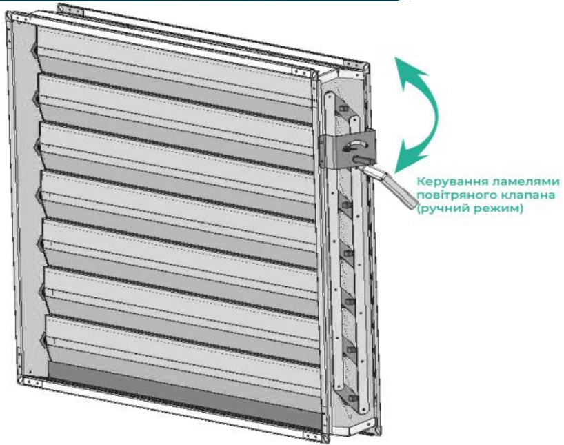
Рисунок 18 Повітряний клапан
