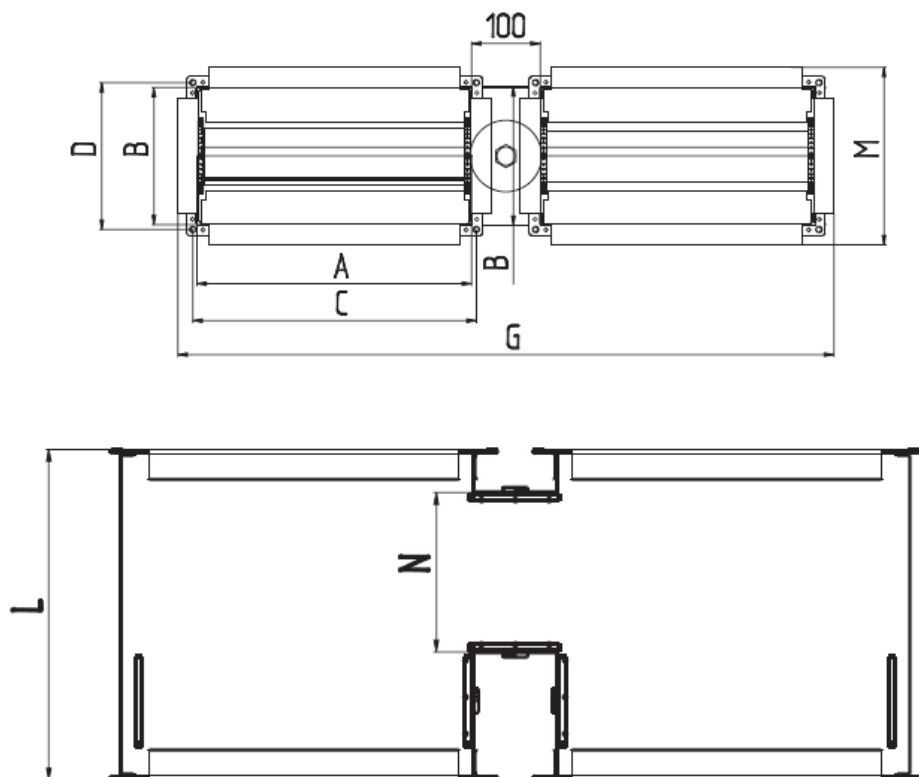
Рисунок 2 – Габаритные и присоединительные размеры
